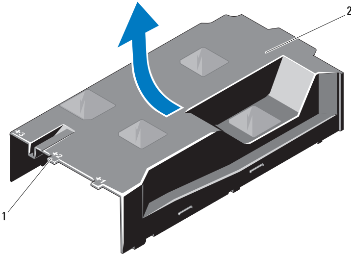
Abbildung 3-4. Kühlgehäuse entfernen und installieren
